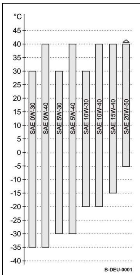
Fig. 153: Diagrama de viscosidad de aceites
